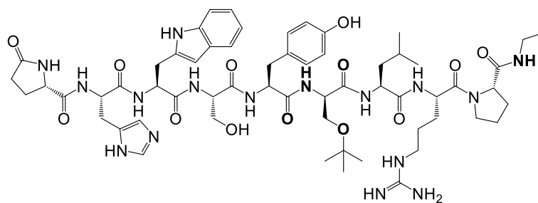
Pyr-His-Trp-Ser-Tyr-D-Ser(tBu)-Leu-Arg-Pro-NHEt
