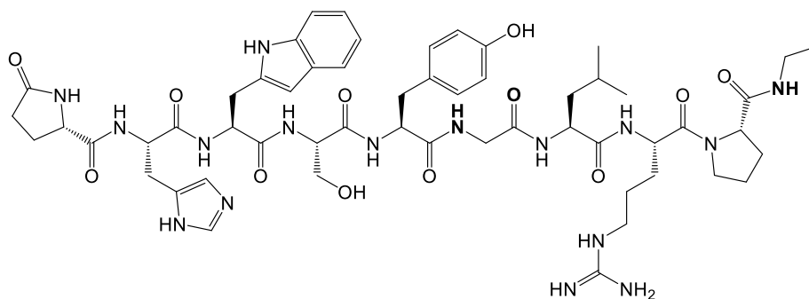
Pyr-His-Trp-Ser-Tyr-Gly-Leu-Arg-Pro-NHEt
