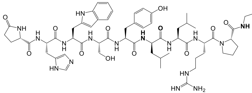
Pyr-His-Trp-Ser-Tyr-D-Leu-Leu-Arg-Pro-NHEt
